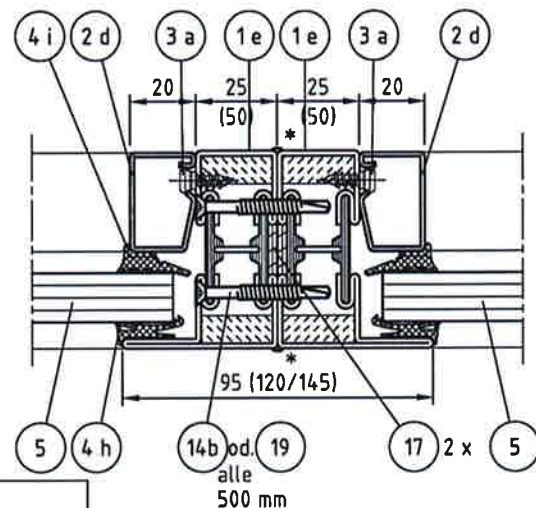
Schnitt D-D
