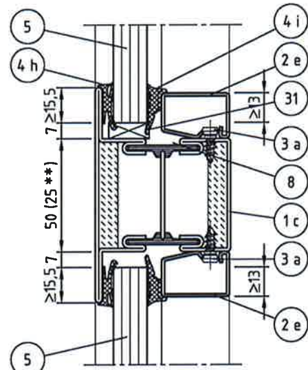
Schnitt B-B
