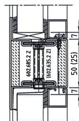
Entwässerungsstülle aus Kunststoff Art. 450.044 und Aluminium Art. 450.042 u. 450.043
