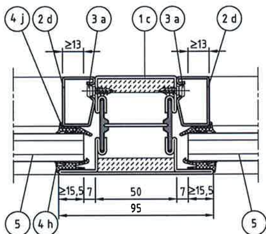
Schnitt C-C
