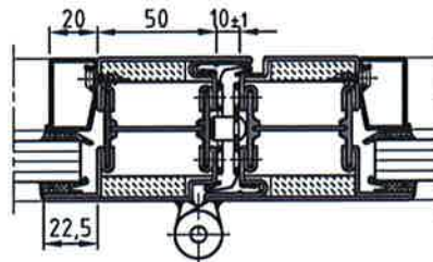
Schnitt E-E
