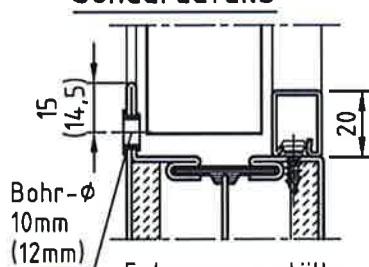
Entspannungsstülle aus Zinkdruckguss Art. 450.046 u. (450.047)
