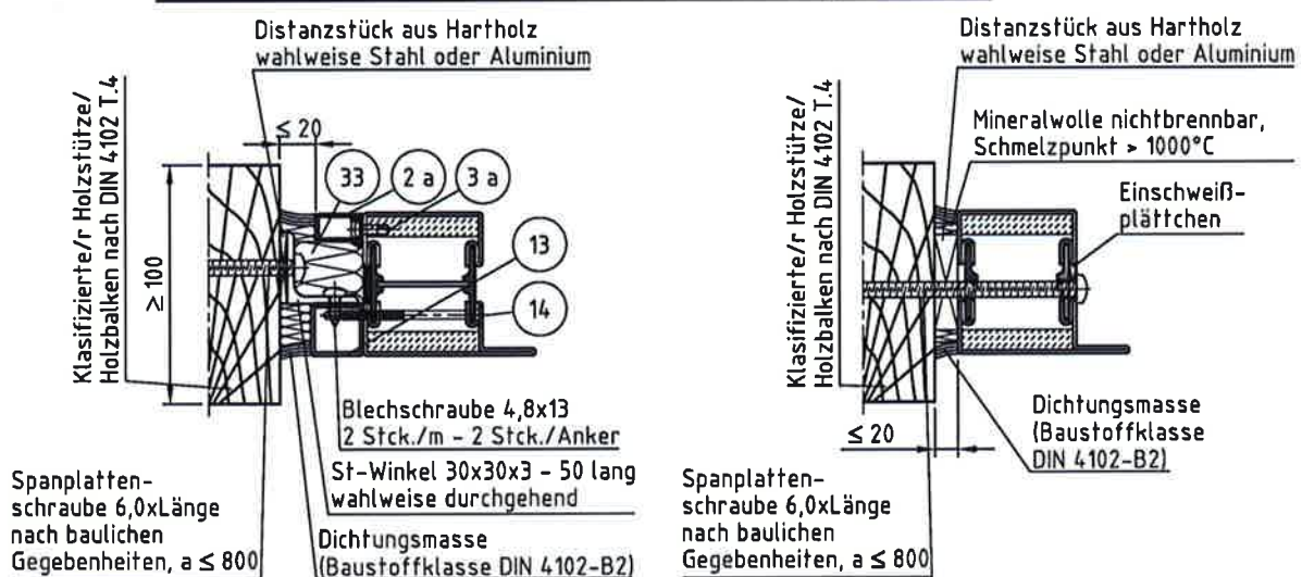
Anschluss an klassifizierte Holzbauteile F30-B nach DIN 4102, Teil 4 ... Seitlicher und oberer Anschluss - Ausführung wahlweise
