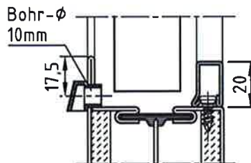
Entspannungsstülle aus Kunststoff
