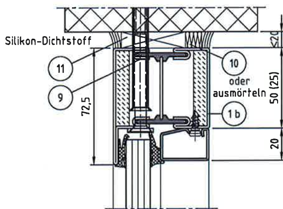
Schnitt A-A , wahlweise
