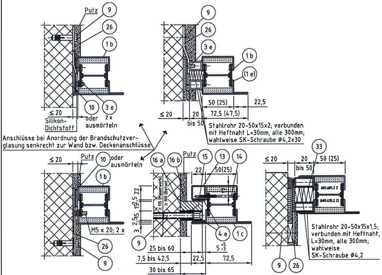
Anschluss an klassifizierte Holzbauteile F30-B nach DIN 4102, Teil 4 ... Seitlicher und oberer Anschluss - Ausführung wahlweise
