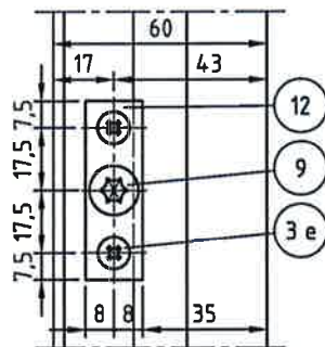
Befestigung wahlweise mit Platte
